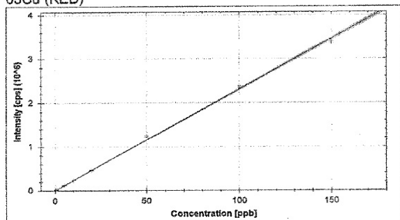
63Cu (KED)
