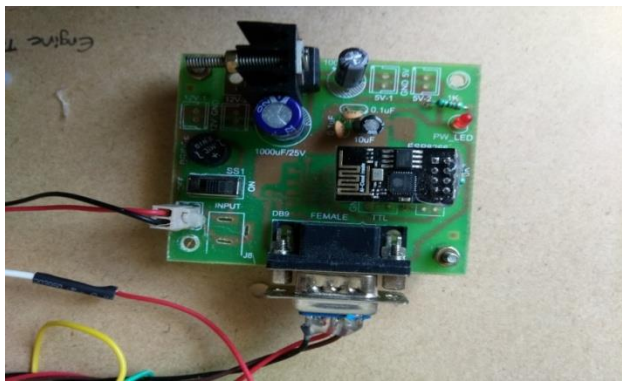
Fig 6 ESP 8266 Wi-Fi module
