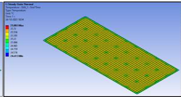
Fig 4. EVA Layer
