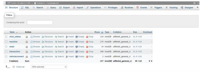
Fig. 15. MySQL Database
