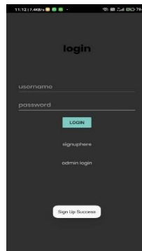
fig 1.2 login page
