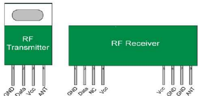
Fig. 5. RF Module devices[9].
