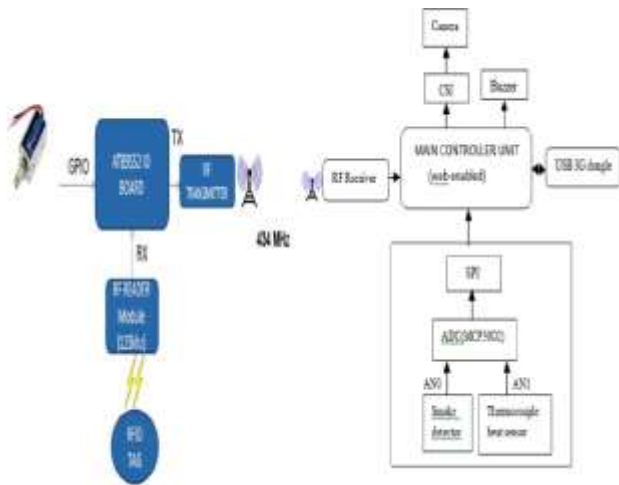
Fig. 1. Function Diagram.
